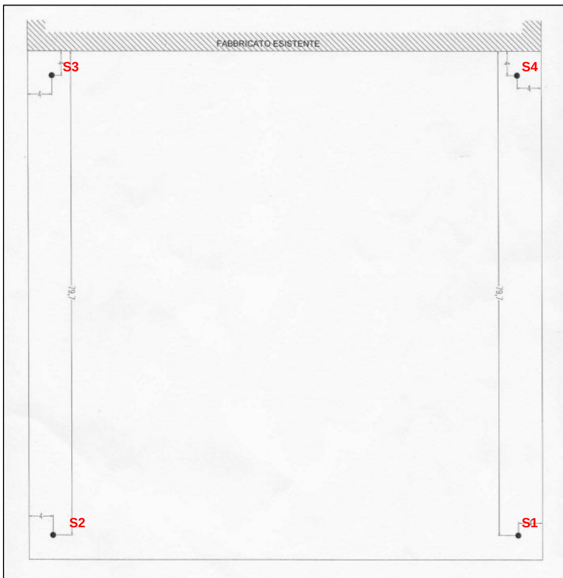
Fig.2 – Ubicazione indagini
